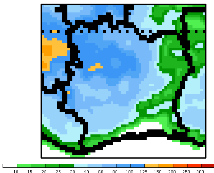
Figure 10 : prévision de la pluviométrie du 22 au 29 Juillet 2019 (source : NOAA, climat Prédiction Center)
