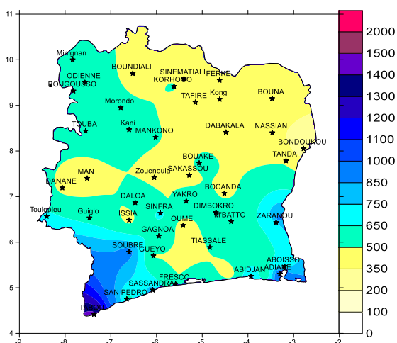
Fig 3 : Cumul pluviométrique (mm) du 1 Janvier au 20 Juillet 2019
