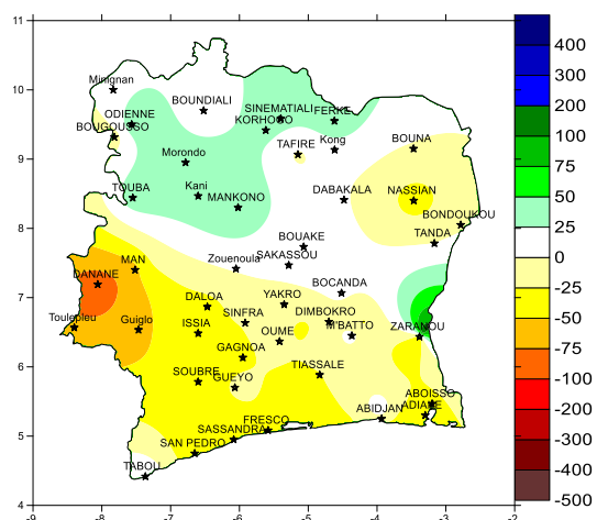
Fig2 : Ecart entre la pluviométrie (mm) du 11 au 20 Juillet 2019 et du 11 au 20 juillet de la normale (1981-2010)
