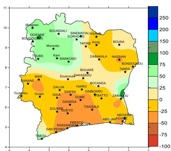
Fig. 9 : Bilan hydrique climatique (mm) du 11 au 20 Juillet 2019
