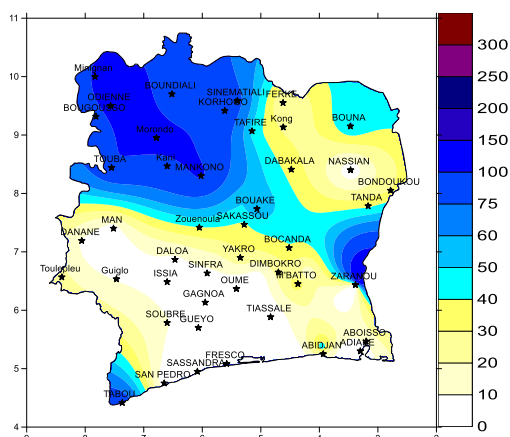
Fig1 : Pluviométrie totale (mm) du 11 au 20 Juillet 2019
