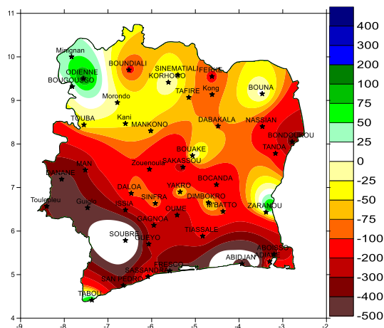
Fig. 4 : Ecart entre Cumuls pluviométriques du 1 Janvier au 20 Juillet 2019 et du 1 Janvier au 20 Juillet de la normale (1981-2010)
